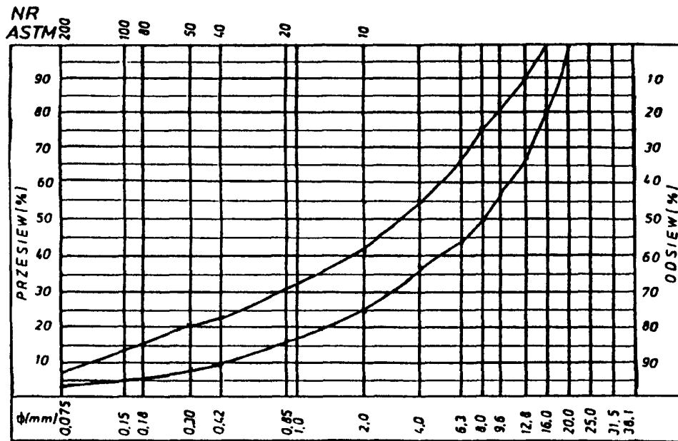
Krzywe graniczne uziarnienia mieszanki mineralnej \phi \leq 20 mm do warstwy wiążącej, wyrównawczej i wzmacniającej z betonu asfaltowego dla KR 3-6
