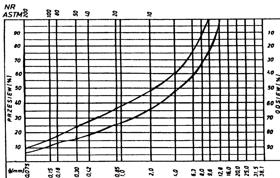
Krzywe graniczne uziarnienia mieszanki mineralnej 0p12,8 mm do warstwy ścieralnej z betonu asfaltowego dla KR 3-6
