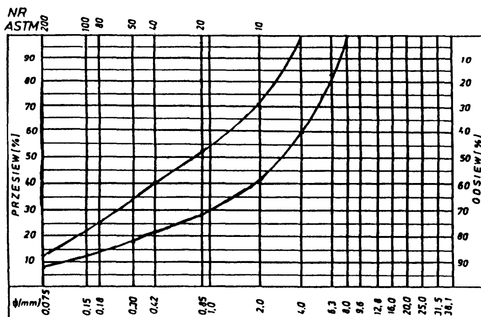
Krzywe graniczne uziarnienia mieszanki mineralnej \phi 8, \phi 6,3 mm do warstwy ścieralnej z betonu asfaltowego dla KR 1-2
