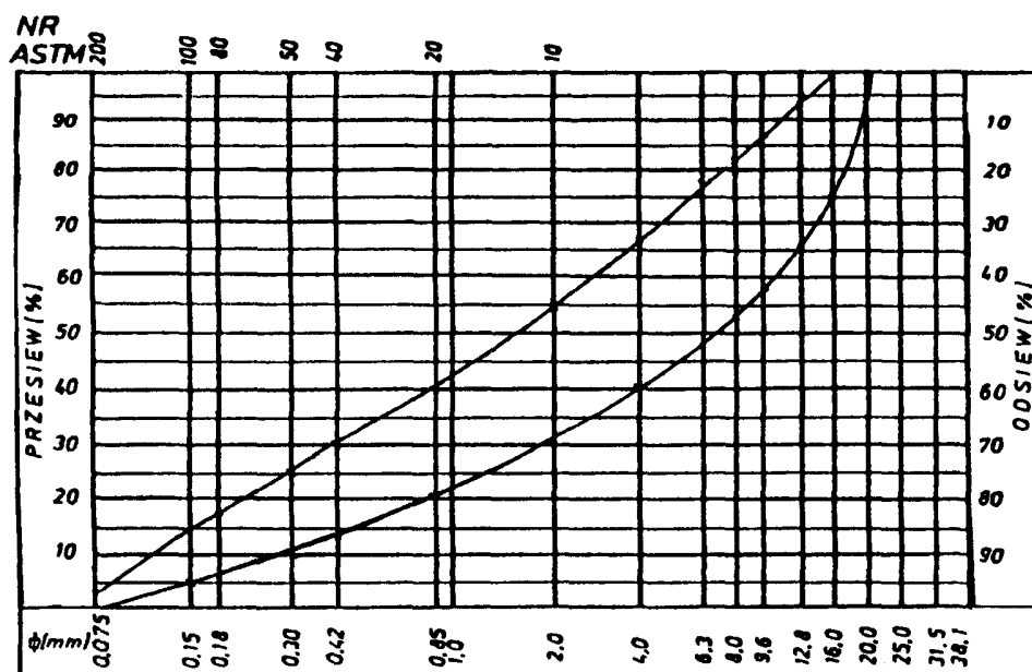
Krzywe graniczne uziarnienia mieszanki mineralnej 0p20 mm do warstwy wiążącej, wyrównawczej i wzmacniającej z betonu asfaltowego dla KR 1-2
