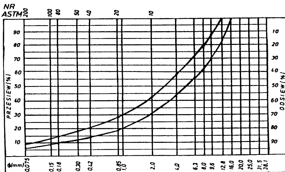
Krzywe graniczne uziarnienia mieszanki mineralnej 0p16 mm do warstwy ścieralnej z betonu asfaltowego dla KR 3-6
