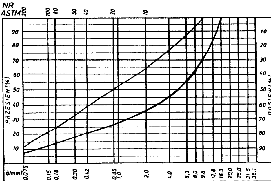
Krzywe graniczne uziarnienia mieszanki mineralnej \phi 16, \phi 12,8 mm do warstwy ścieralnej z betonu asfaltowego dla KR 1-2
