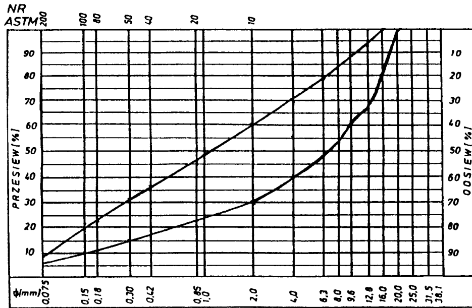
Krzywe graniczne uziarnienia mieszanki mineralnej \phi 20 mm do warstwy ścieralnej z betonu asfaltowego dla KR 1-2
