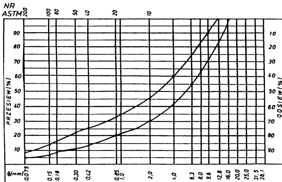
Krzywe graniczne uziarnienia mieszanki mineralnej \phi \leq 16 mm do warstwy wiążącej, wyrównawczej i wzmacniającej z betonu asfaltowego dla KR 3-6
