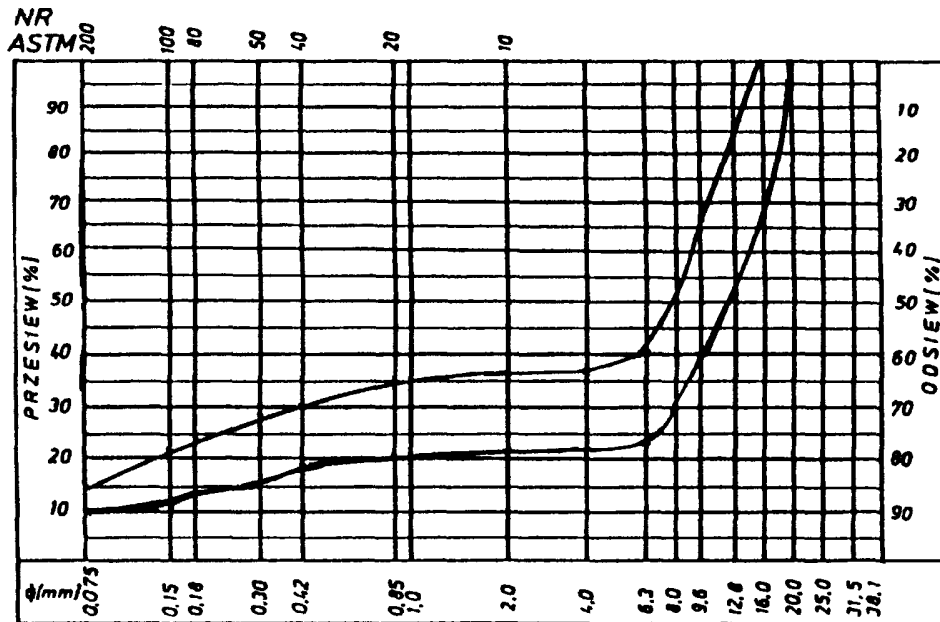
Krzywe graniczne uziarnienia mieszanki mineralnej 0p20 mm o nieciągłym uziarnieniu do warstwy ścieralnej z betonu asfaltowego dla KR 3-6
