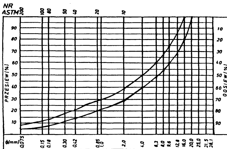
Krzywe graniczne uziarnienia mieszanki mineralnej \phi 20 mm do warstwy ścieralnej z betonu asfaltowego dla KR 3-6
