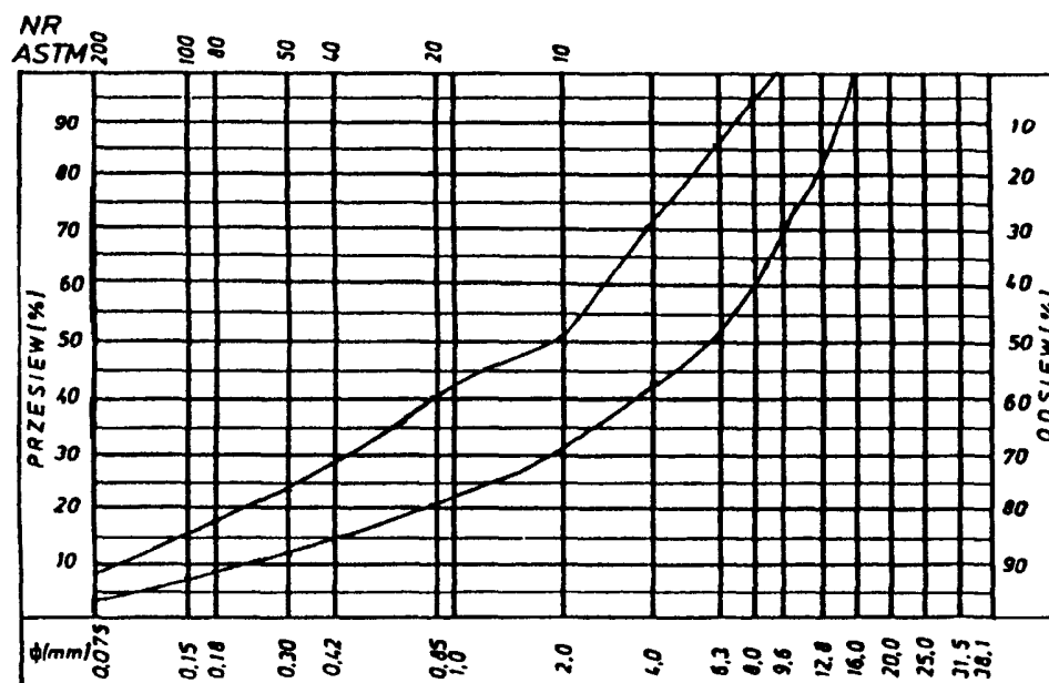
Krzywe graniczne uziarnienia mieszanki mineralnej 0p16 mm do warstwy wiążącej, wyrównawczej i wzmacniającej z betonu asfaltowego dla KR 1-2
