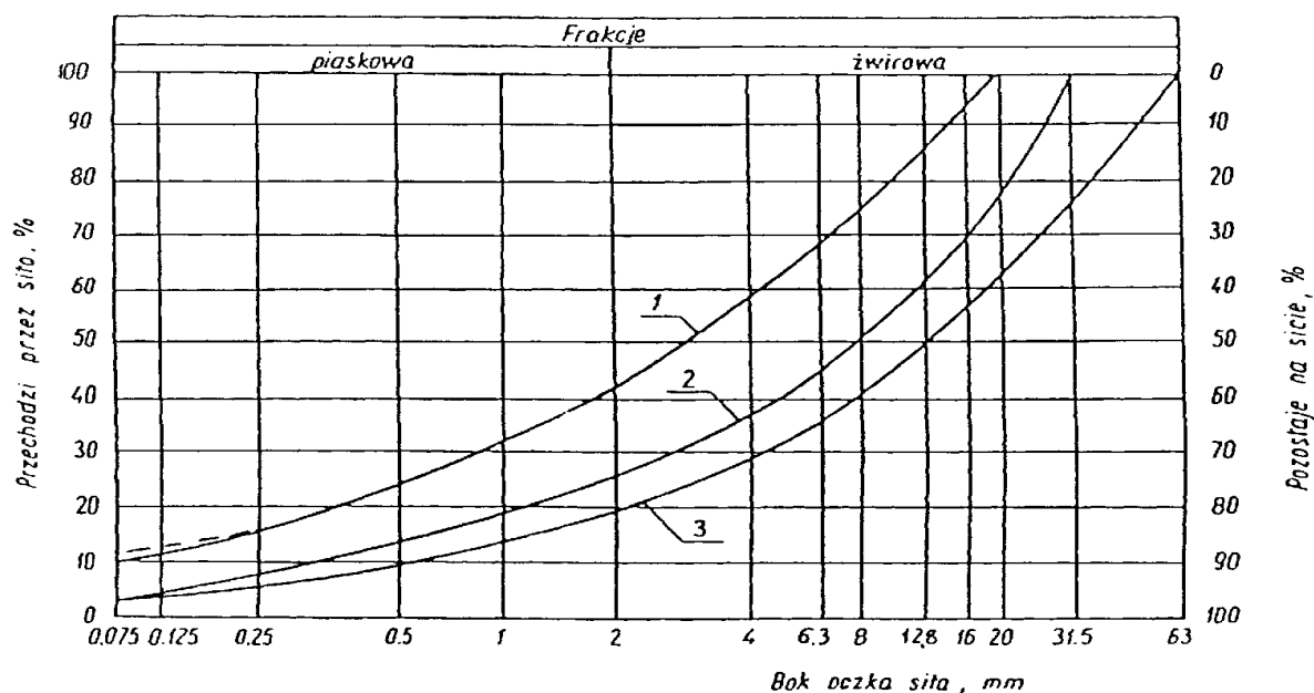
Rysunek 1. Pole dobrego uziarnienia kruszywa przeznaczonych na podbudowę wykonywane metodą stabilizacji mechanicznej
